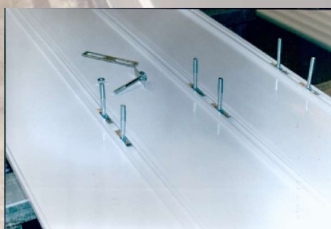
Introducir tornillo con chapa de agujero cuadrado en ranuras
